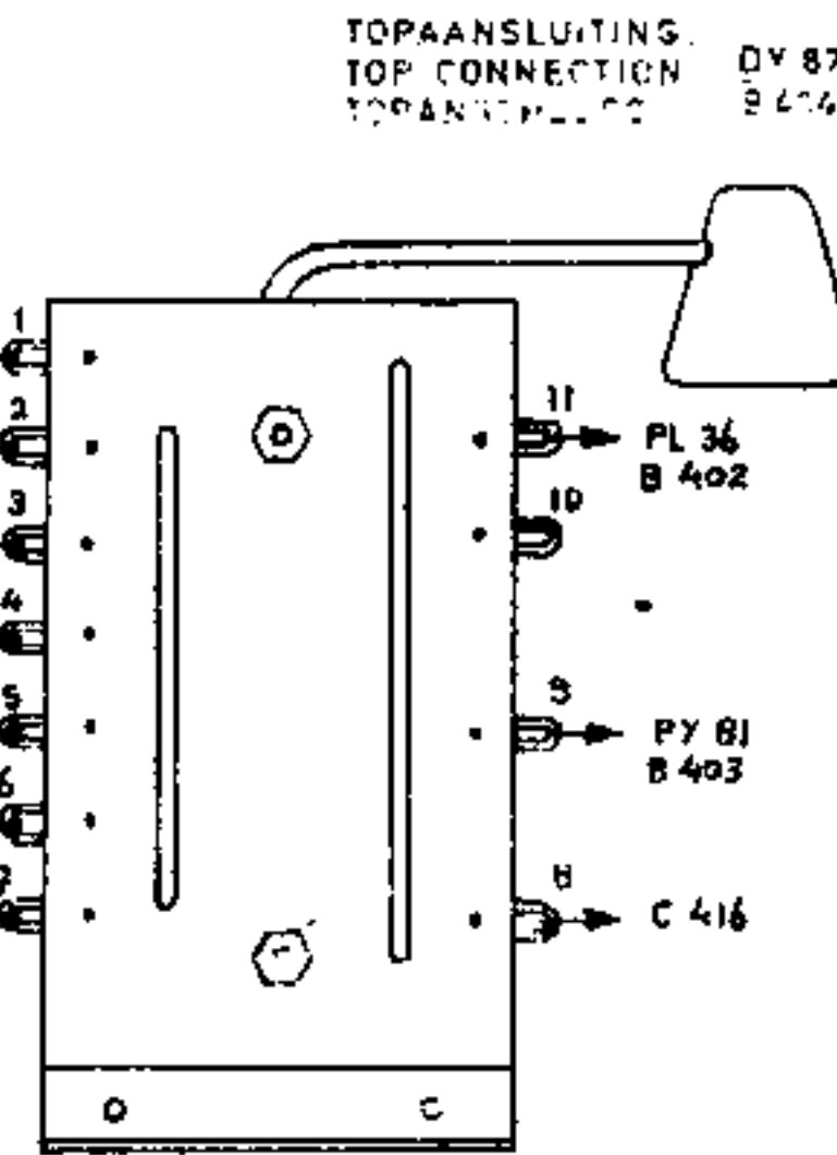
LIJNUITGANGS TRAFU LINE OUTPUT TRANSF. ZEILENAUSG. ÜBERTRAGER AT 2018/20 : TV 5625 C
