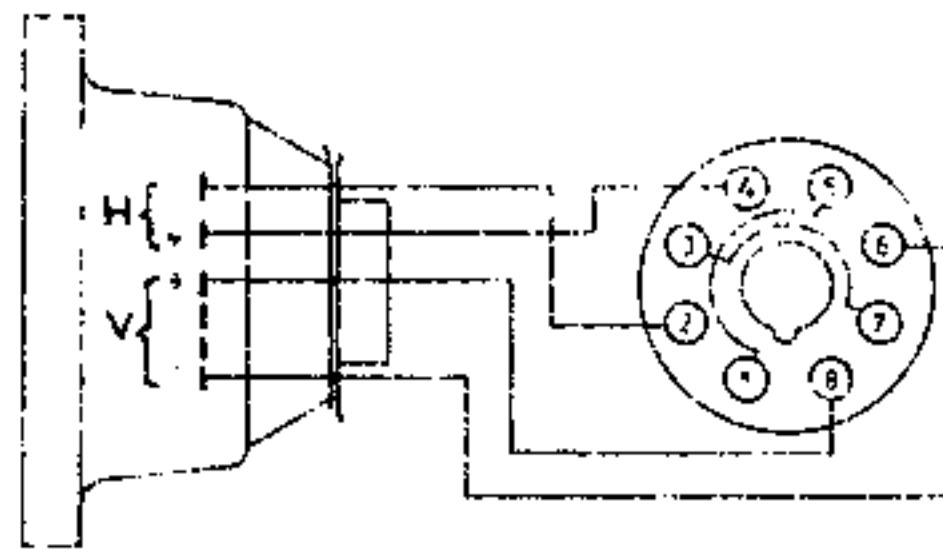
DEFLECTIE JUK DEFLECTION YOKE ABLENKEINHEIT AT 1005/02
